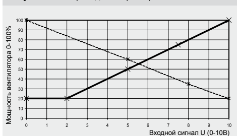
Рисунок 22 – Переводная характеристика ОХА
