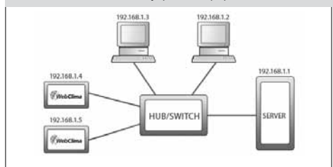
Рис. 8 – WebClima на внутренней фирменной сети
