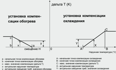
Рис. 21б – пояснения и настройка компенсации
