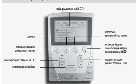
Рис. 38 – пульт управления HMI
