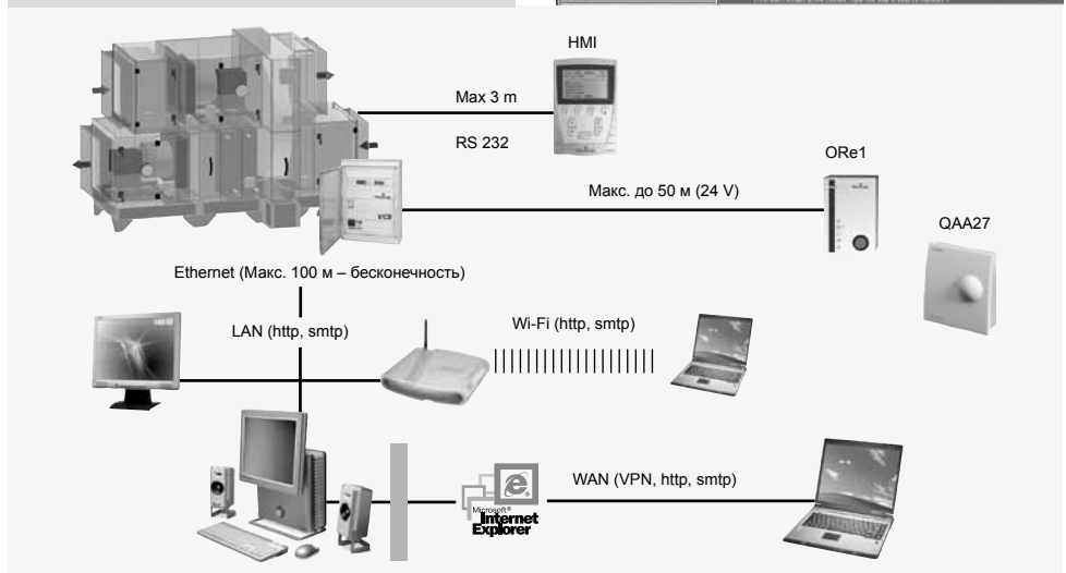
Рис. 3 – пример комплексного доступа к оборудованию
