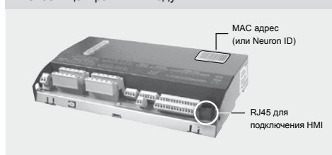
Рис. 39 – центральный модуль
